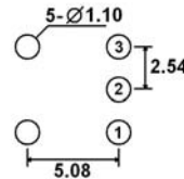
C - SPDT
