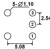
C - SPDT
