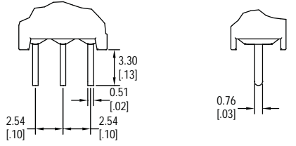
C SPDT
