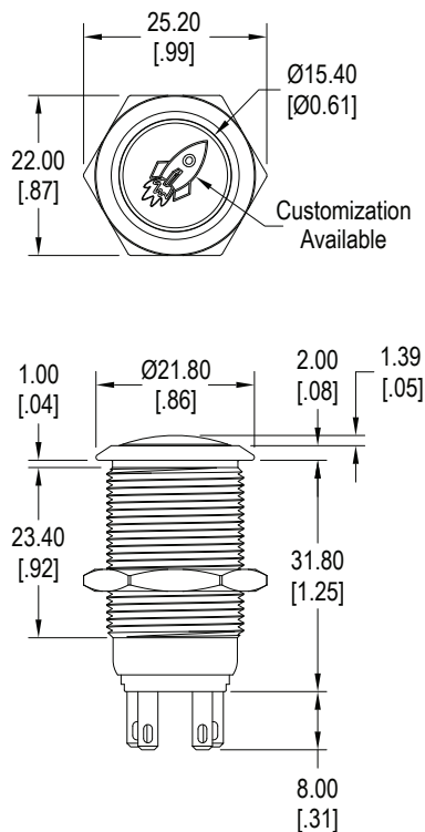
EC Actuator
