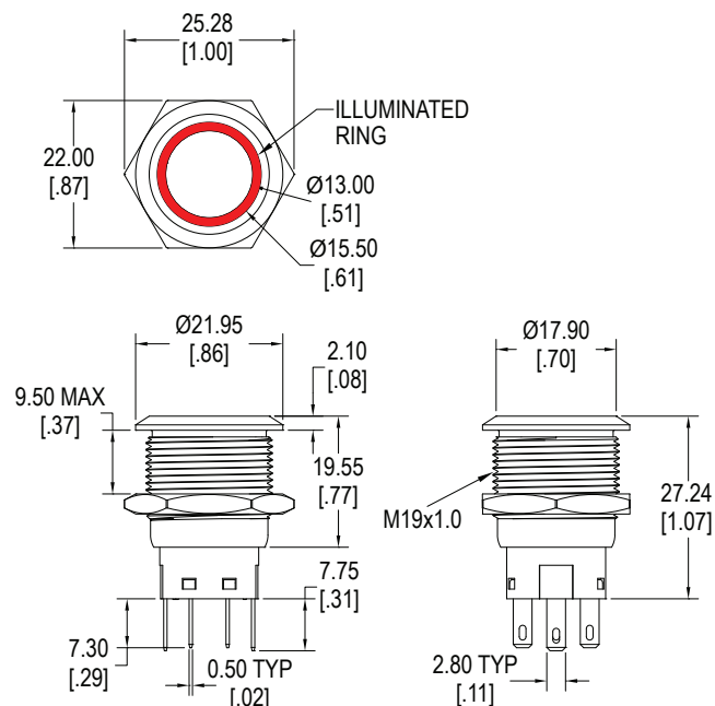
K Actuator
