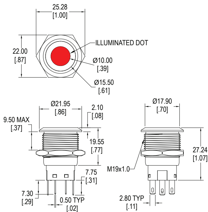
C Actuator
