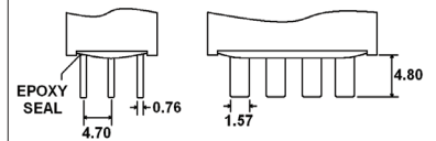
D, 4 pole
