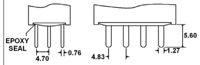
C, 4 pole
