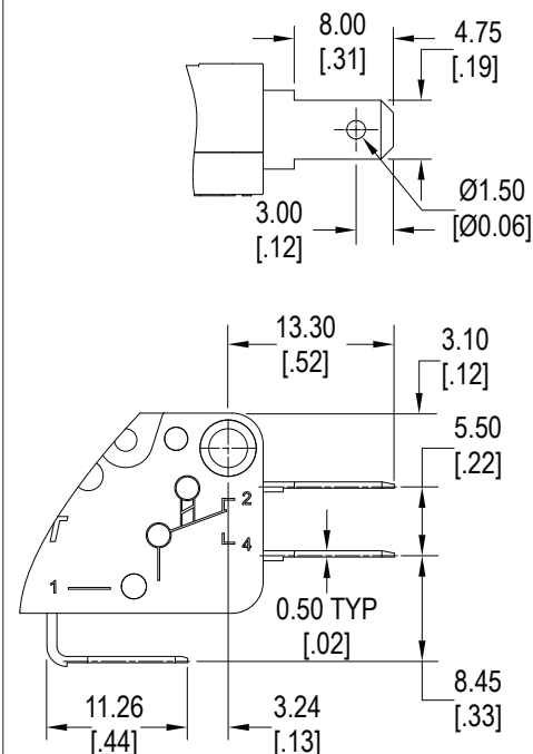
SPDT
