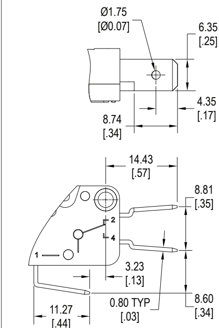
SPDT
